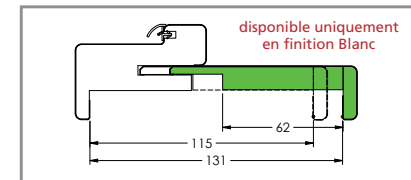
Extension de 62 pour cloison finie de 115 à 131 mm
