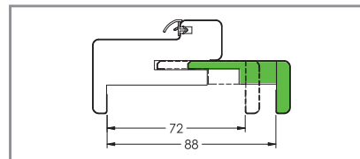
Extension de 19 pour cloison finie de 72 à 88 mm
