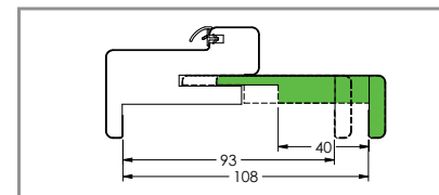
Extension de 40 pour cloison finie de 93 à 108 mm
